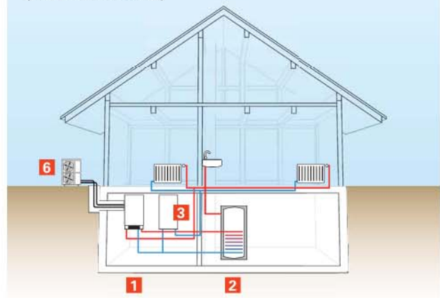
Wärme aus der Luft (mit Außeneinheit)
